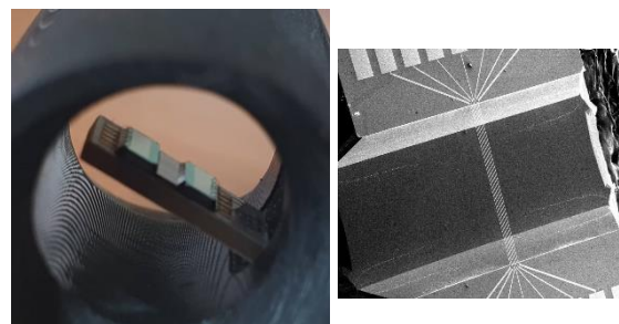
Fig. 6. Flow sensor WA
